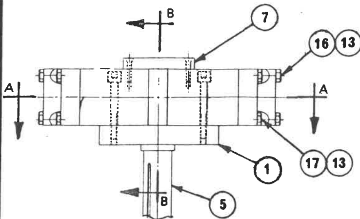
PIVOT HYDRAULIQUE POUR ROTATION 90° (192-1127-001-00-4) (HYDRAULIC PIVOT DEVICE 90° ROTATION)
