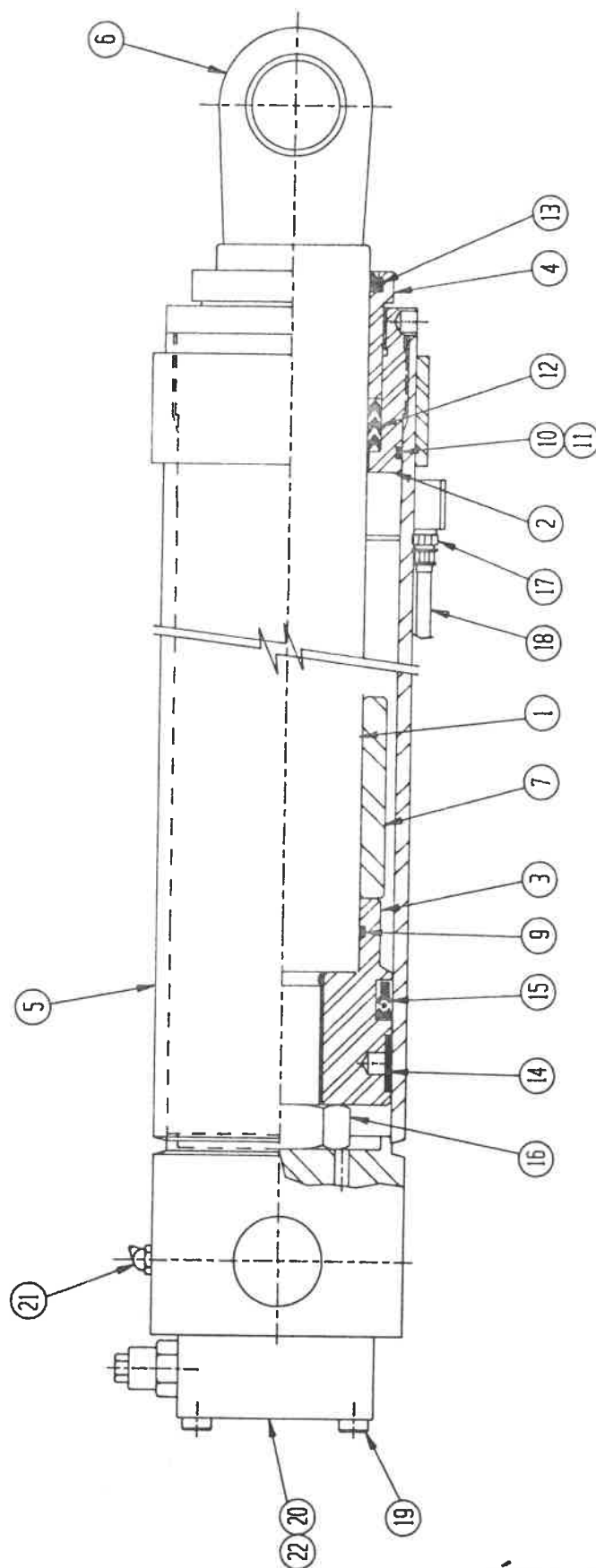
VÉRIN ASS'É (STABILISATEUR (CYLINDER ASS'Y) (500-9081-001-01-4)
